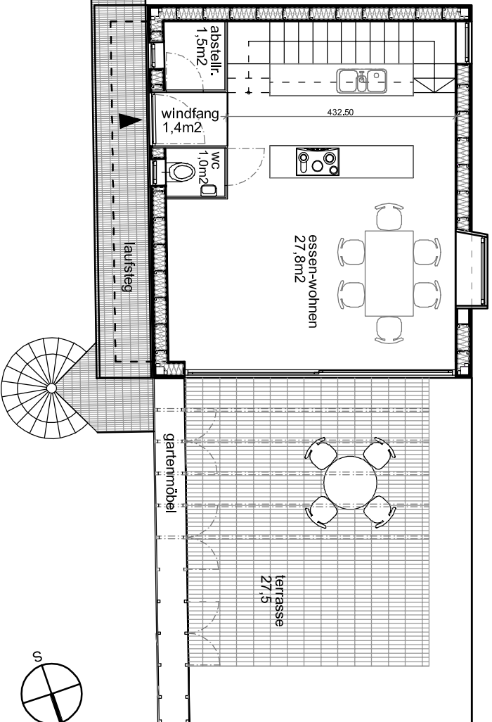
wohn aptman 11
